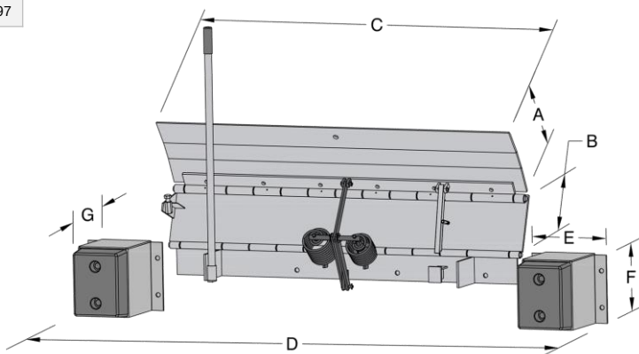
Isométrico Mini Dock
